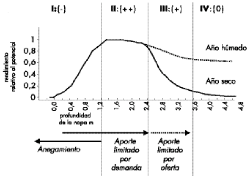
Figura 1: Función de respuesta de los rendimientos a la profundidad de napa. Los rendimientos se expresan como valores relativos al potencial que puede obtenerse cuando no hay limitaciones hídricas.
